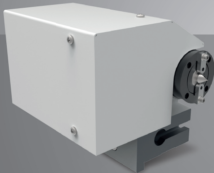
POUPÉE PORTE-PIÈCE avec pointe non entraînée (pointe sèche)
